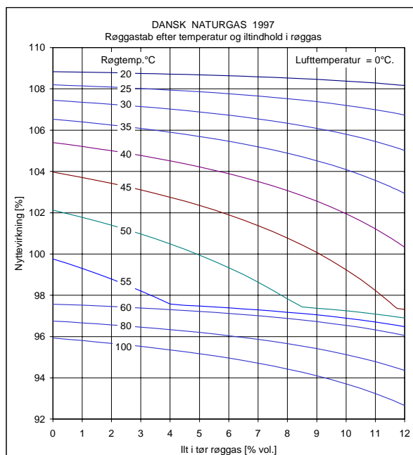
Figur 5 Beregnet nyttevirkning
