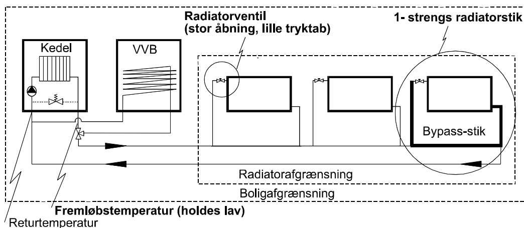
Figur 1 Opbygning af et 1-strengs anlæg med energibalancer
