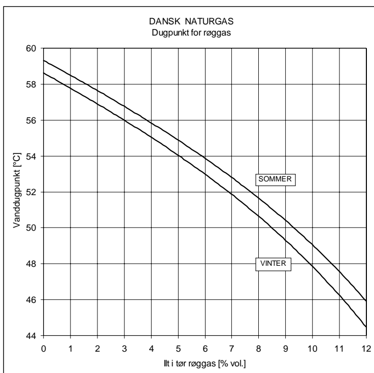
Figur 3: Her ses iltprocentens betydning for røggassernes dugpunkt og dermed kedlens evne for kondensering
