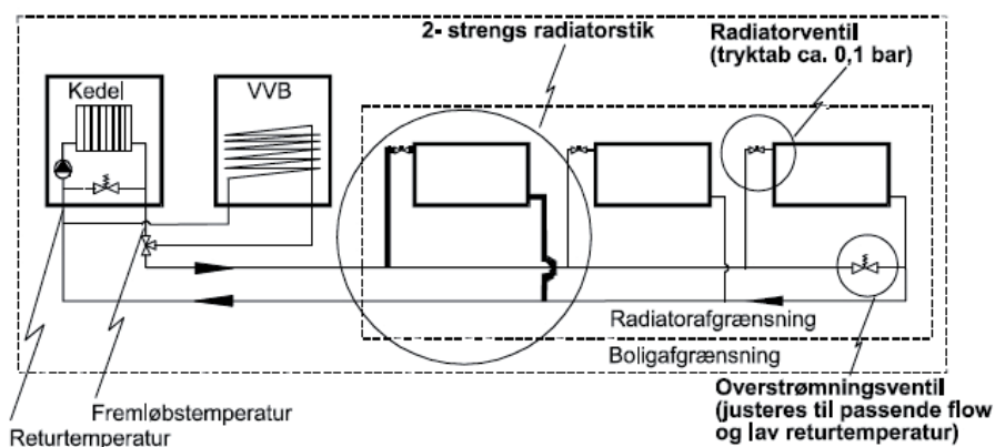
Figur 1 Opbygning af et 2-strengs anlæg med energibalancer
