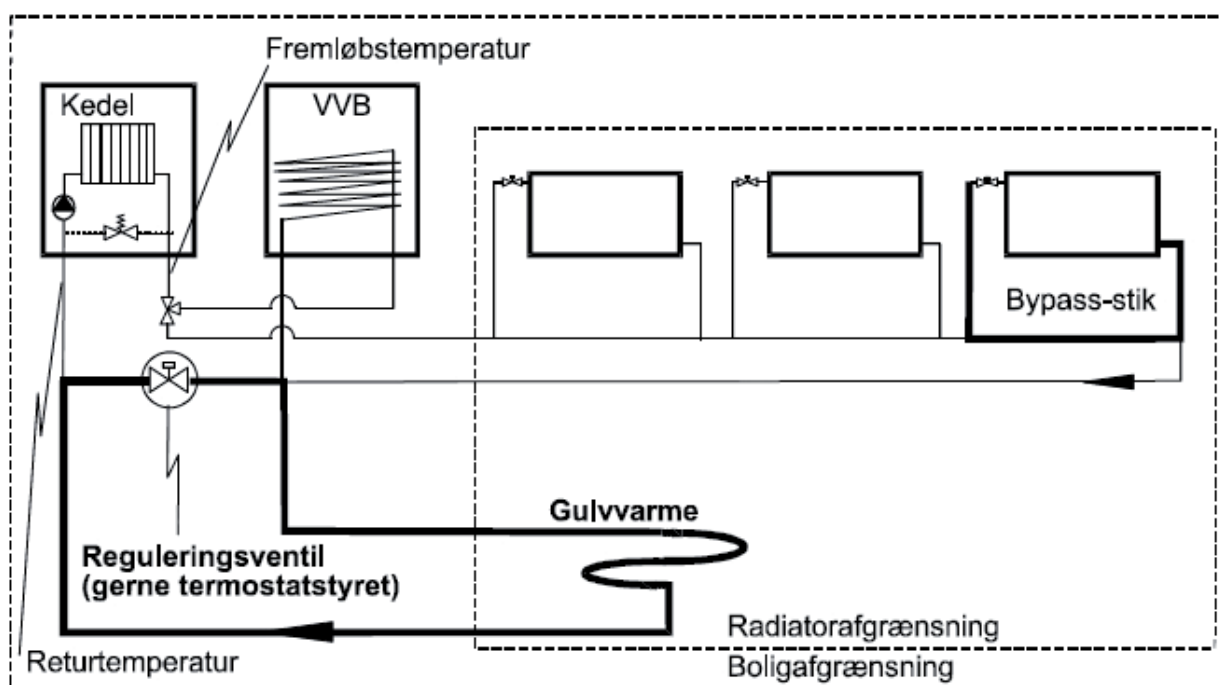
Figur 4: 2-strengs anlæg kombineret med gulvvarme og dermed optimal afkøling af returvandet
