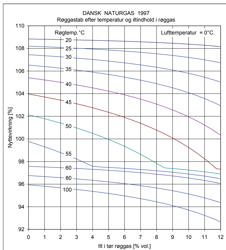
Figur 5 Beregnet nyttevirkning
