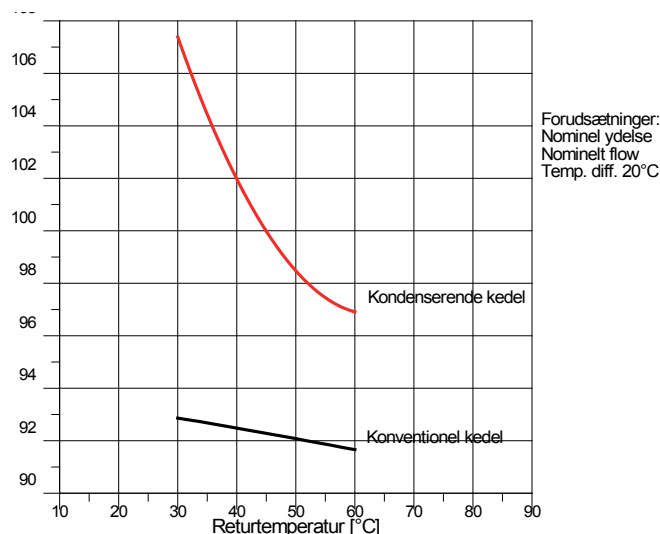
Figur 2 Beregnet nyttevirkning som funktion af returtemperaturen
